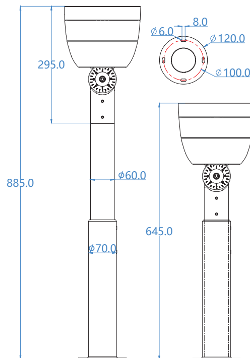
Телескопическая опора
